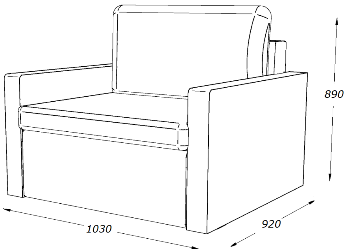
Функциональные размеры.
